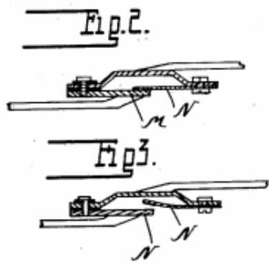
1912 Limitatore in lega fusibile Hoffmann per coperta di riscaldamento (US Patent 1096916). La lega fusibile salda insieme le lame M e N.
