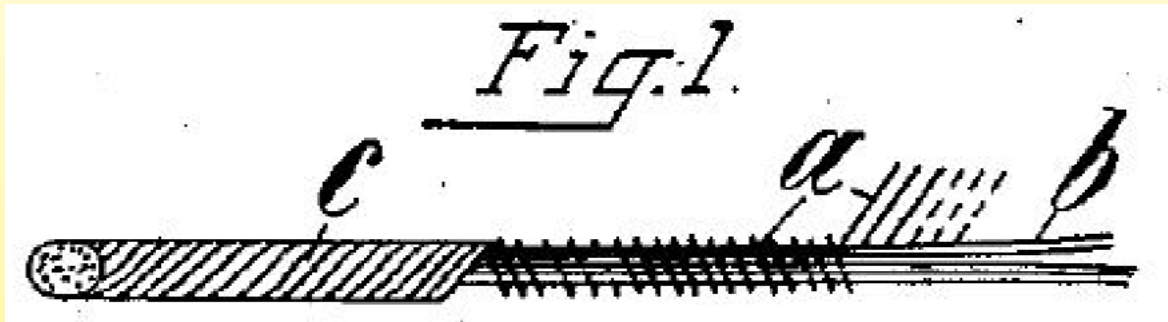
Cavo scaldante (brevettato da Camille Herrgott, 1901). A = filo scaldante; B = anima tessile; C = involucri esterno avvolto in direzione opposta al filo scaldante.
