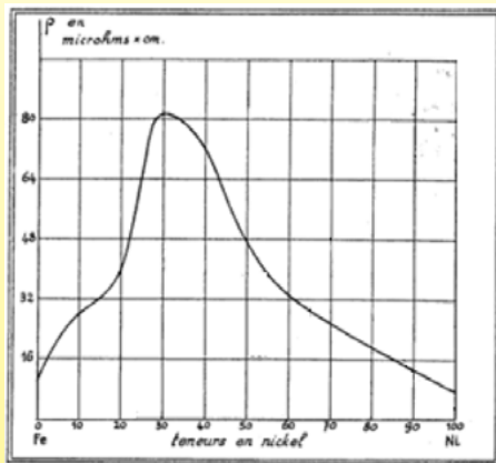
Variatione della resistività: curva rispetto al contenuto di nichel nelle leghe ferro-nichel (La Nature, 1934, Nickel alloys and their applications, P215)
