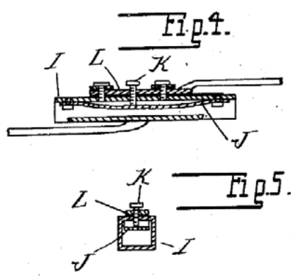
1912 Termostato bimetallico Hoffmann per coperta riscaldante (US Patent 1096916) J è una lama bimetallica rivettata a entrambe le estremità. Si suppone che il contatto elettrico si apra tra la lama J, che si deforma quando la temperatura aumenta, e la vite di regolazione K.
